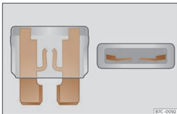
Billede 182 Sikring, der er brændt over
