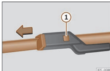
Billede 173 Udskiftning af viskerblade foran
