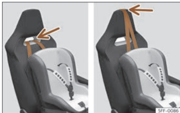
Billede 42 Passagersæde: indstilling og montering ved anvendelse af Top Tether-rem
