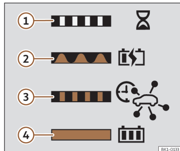
Billede 60 På indersiden af batteriladeklappen: mærket med informationer vedr. opladningsindikatoren
