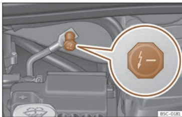
Billede 175 I frontrummet: starthjælpspunkt (stelforbindelse)
