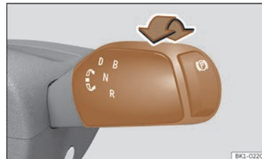
Billede 106 Gearvælger med knap til elektronisk parkeringsbremse
