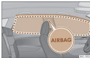
Billede 32 Placering af hovedairbags
