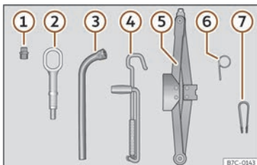
Billede 170 I bagagerummet under bagagerumsbunden: bilens værktøj
