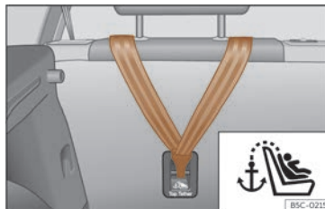
Billede 39 Bagsiden af bagsædet: forankring til Top Tether-fastgørelsesremmen
