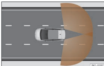
Billede 113 Sensorernes registreringsområde
