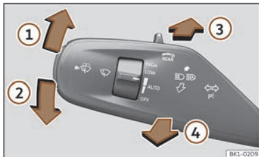
Billede 94 Blink- og fjernlysarm
