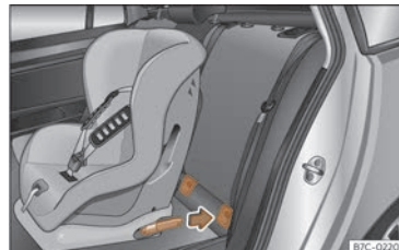
Billede 39 Bagsæde: montering af børnesæde med ISOFIX-system
