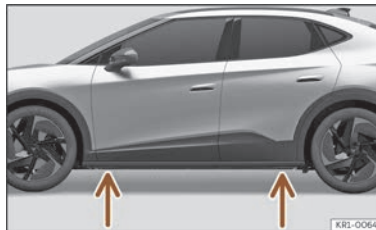
Billede 206 Løftepunkter til donkraften.
