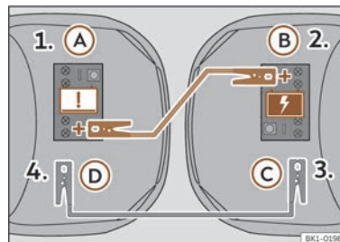
Billede 185 Tilslutningsskema over startkabler
