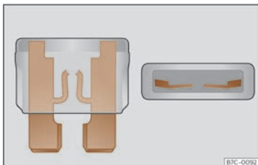
Billede 193 Sikring, der er brændt over
