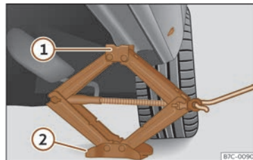
Billede 207 Længdevange: påsætning af donkraft
