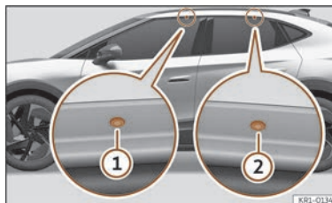
Billede 174 Fastgørelsespunkter til længdevangerne til tagbøjlesystemet
