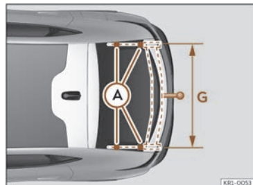
Billede 180 Anhængertræk: mål og fastgørelsespunkter
