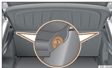
Billede 166 I bagagerummet: af- og påmontering af bagagerumsafdækning
