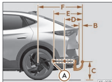
Billede 179 Anhængertræk: mål og fastgørelsespunkter
