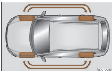
Billede 202 Ombytning af hjul
