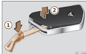
Billede 66 Bilnøgle: åbning af afdækning til batterirum
