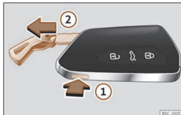
Billede 65 Bilnøgle: udtrækning af nøglekam
