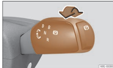
Billede 106 Gearvælger med kontakt til elektronisk parkeringsbremse
