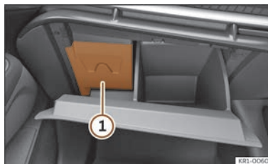
Billede 191 Højrestyret bil: afdækning til sikringsboks i instrumentpanelet i passagersiden
