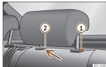
Billede 88 Hovedstøtte bag: afmontering
